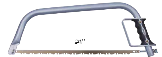
K-6230 Bladlengte: 533mm / 21" Ø 170mm C ⚡ 620 640 Zaagblad: K-6230-1
