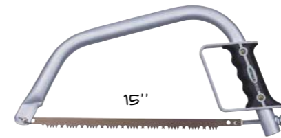
K-6210 Bladlengte: 381mm / 15" Ø 135mm C ⚡ 460 510 Zaagblad: K-6210-1
